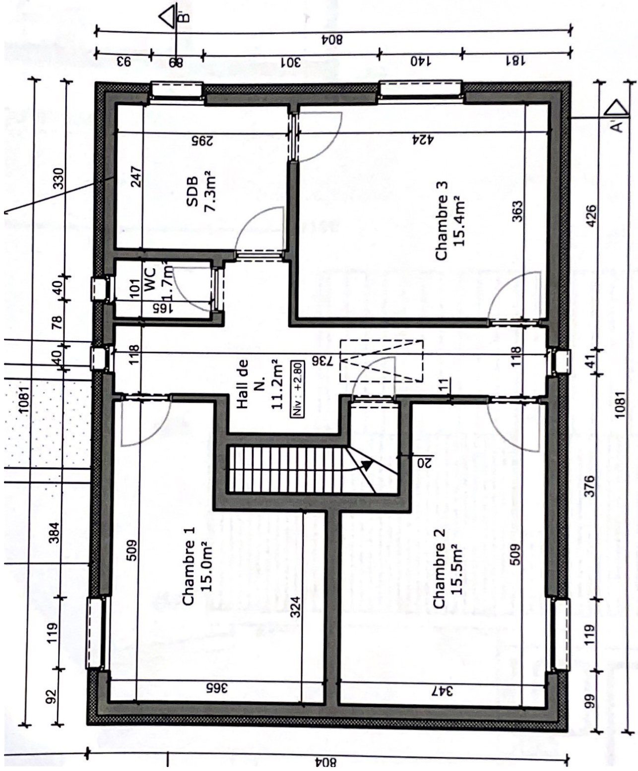
Etage ————— 1/100
